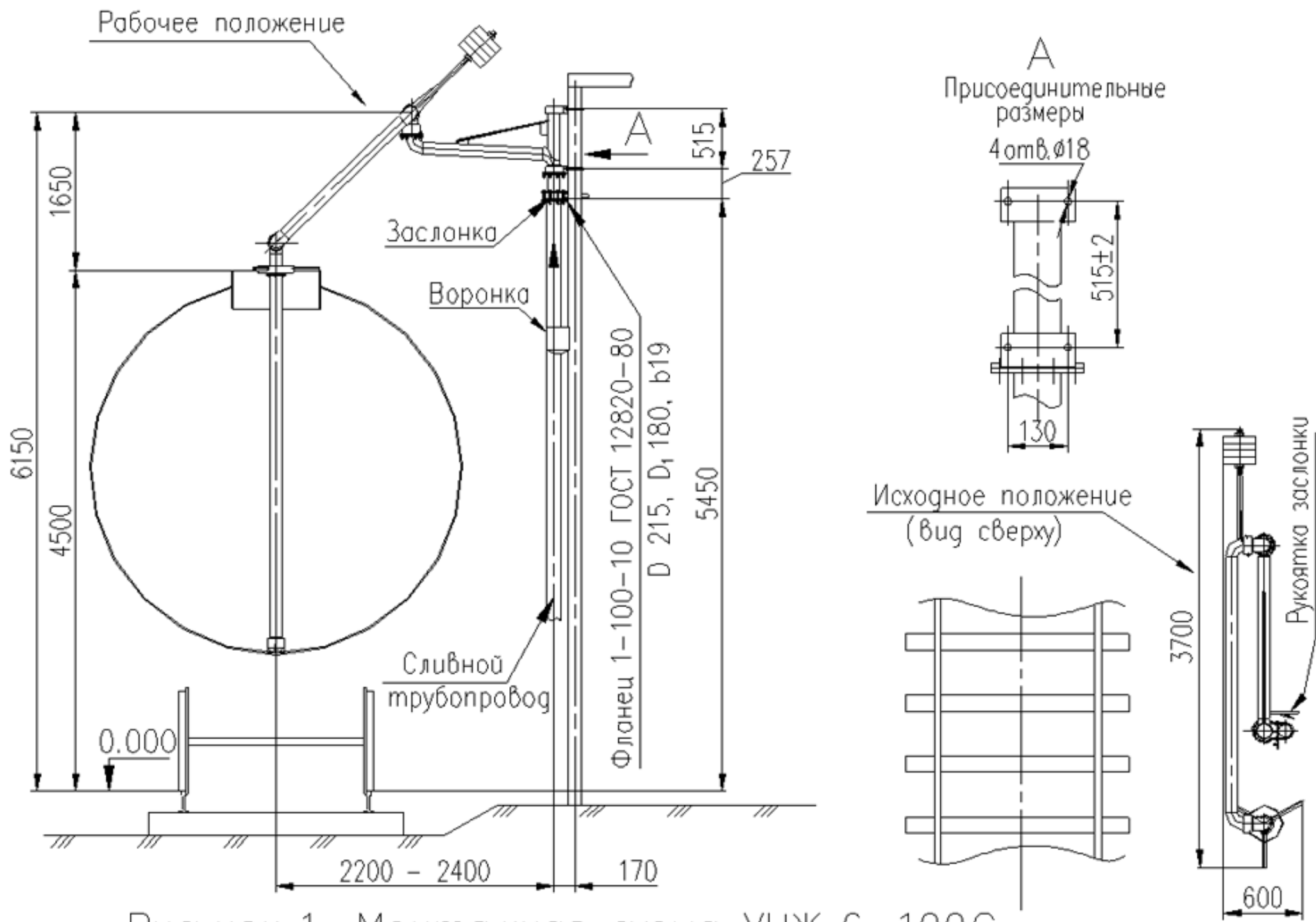
Рисунок 1—Монтажная схема УНЖ 6-100С
