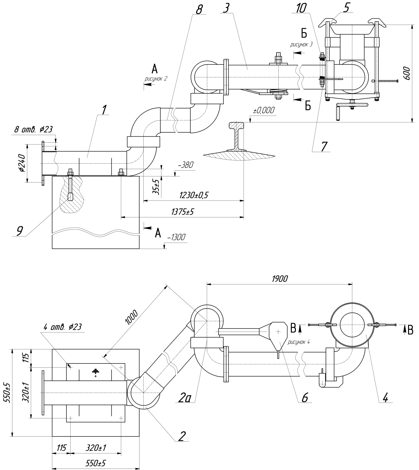
Рисунок 1 – Установка для нижнего слива нефти и нефтепродуктов железнодорожных вагонов-цистерн УСН-150 ХЛ 1
