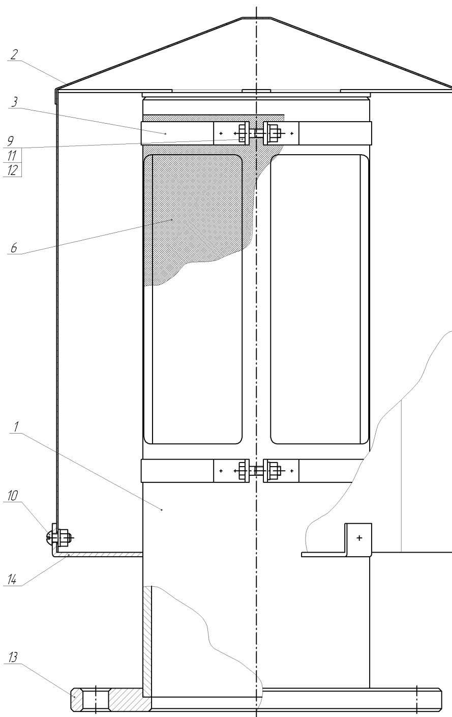
Рисунок 1 – Патрубок вентиляционный ПВ.
