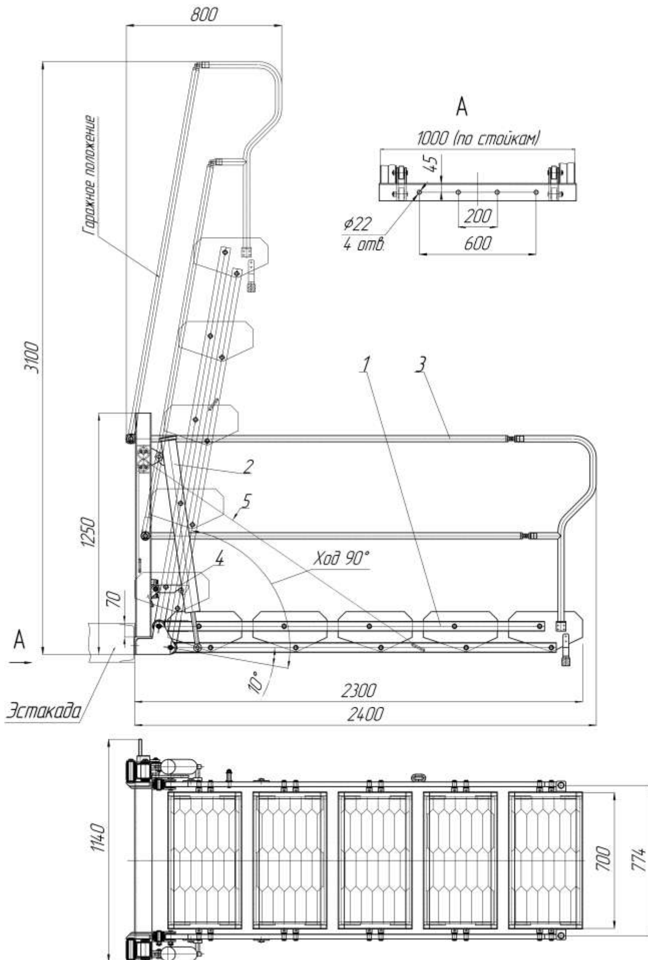
Рисунок 2 – Мостик переходной МПУ-0,7/2,3-5-А
